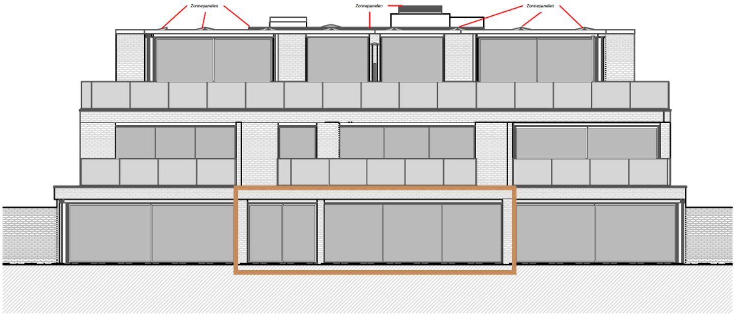
ACHTERGEVEL ZUID
